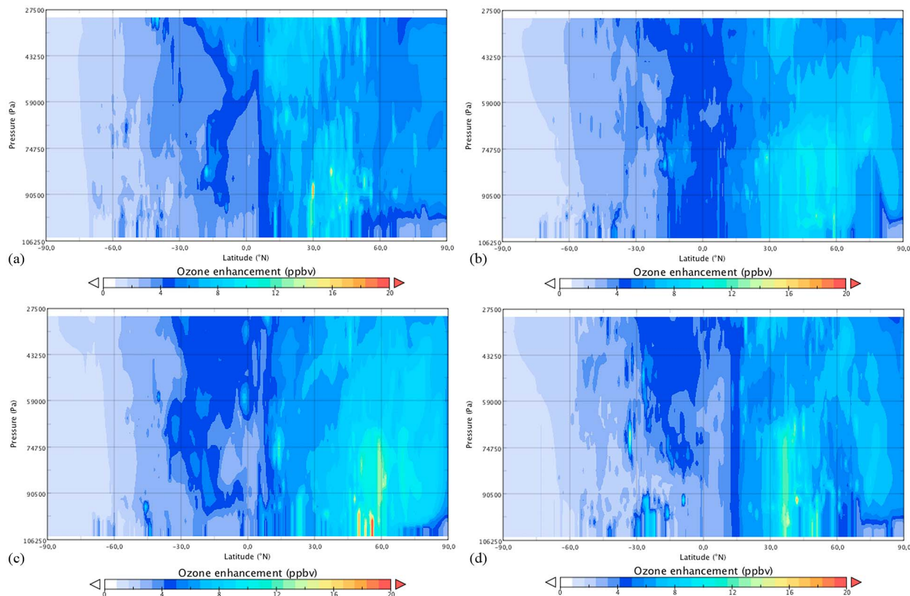
Figure 7. Vertical cross sections of the maximum hourly enhancement concentrations for O 3 at longitude (a) 90W, (b) 30W, (c) 10E, and (d) 130E.
